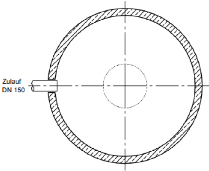
GRUNDRISS
