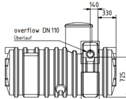
left hand view Ansicht von links
