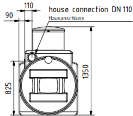
front view Ansicht von vorn
