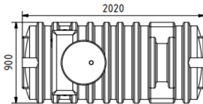
top view Ansicht von oben
