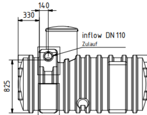
righthand view Ansicht von rechts
