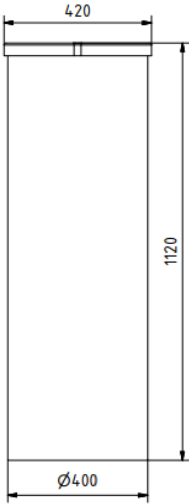
front view Ansicht von vorn
